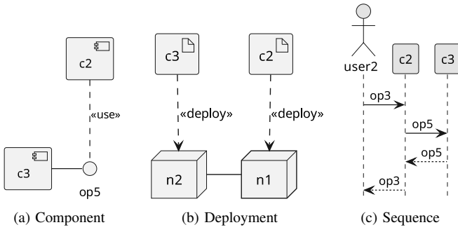
Fig. 1. UML diagrams
